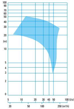
CMX 23... -2 pole
