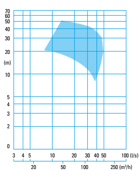
CMX 13... -2 pole
