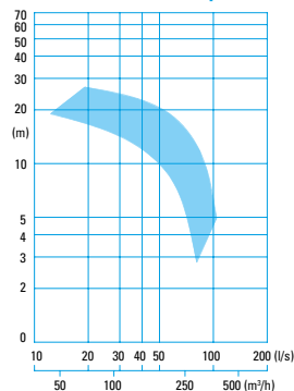
CMX 34... -4 pole
