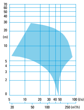
CMX 24... -4 pole
