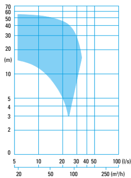
CV 23... -2 pole
