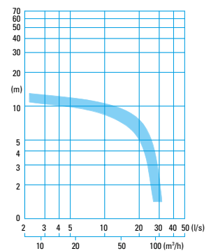
CTP... -4 pole
