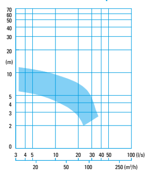
CMX 13... -4 pole
