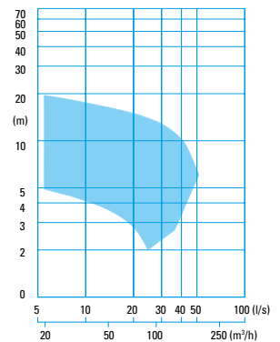
CMX 23... -4 pole
