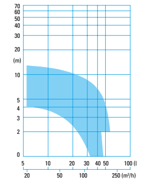
CMX 24... -6 pole
